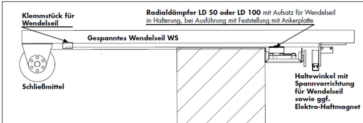
Aufbau und Komponenten des DICTAMAT 50 WS
